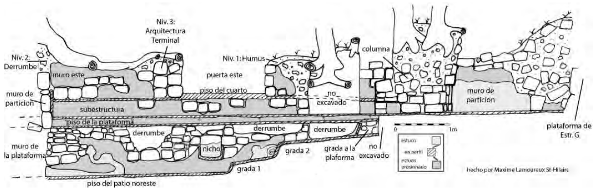
Figura 5.8 Perfil Norte de la Unidad CR20F-8. Cuarto Norte de la Estructura 13Q-4F (Dibujo por M. Lamoureux St-Hilaire)
