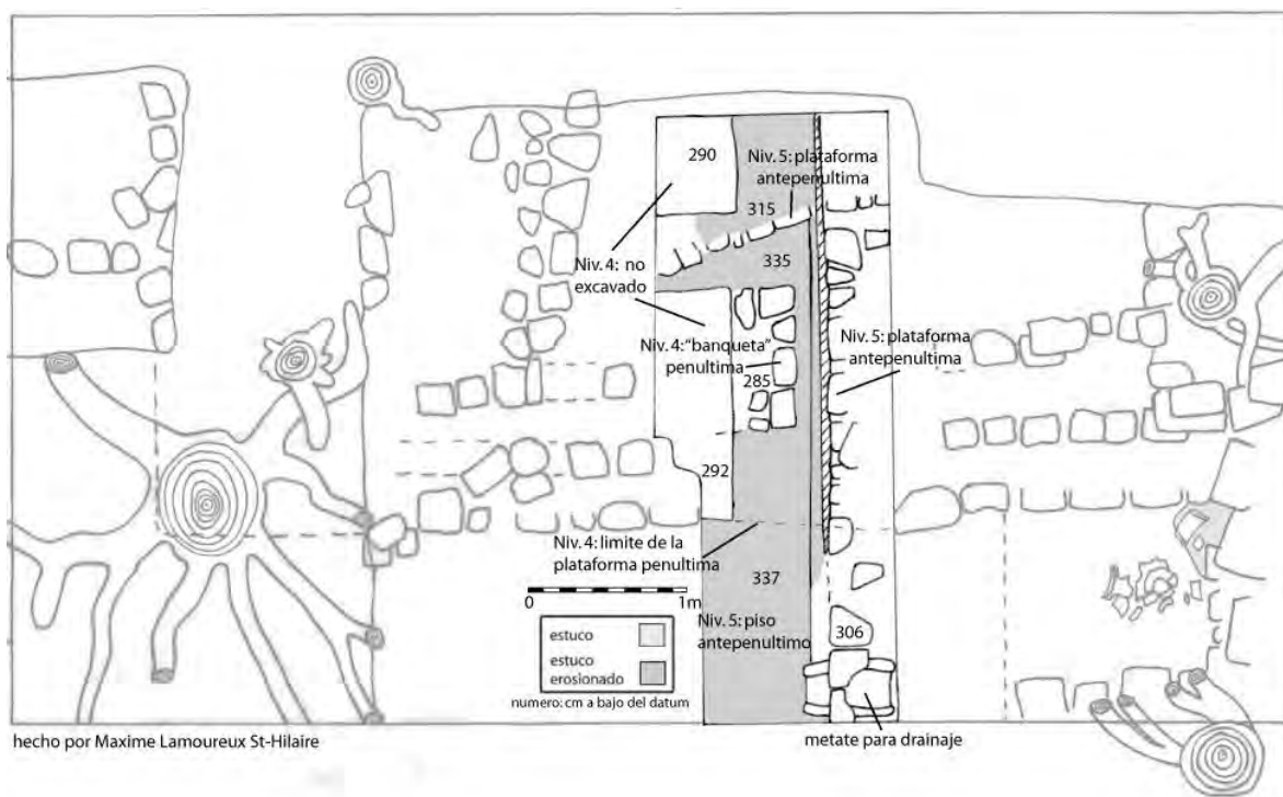
Figura 5.16. Planta superior de la unidad CR20H-1, penúltima y antepenúltima fase arquitectónica de la Estructura 13Q-4H-1 (Dibujo por M. Lamoureux St-Hilaire)
