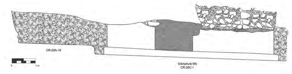
Figura 3.5 Perfil Sur Unidades CR-20C-1 y CR-20A-10 (Dibujo por E. Bustamante)
