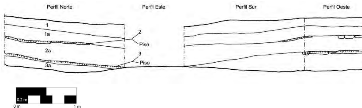
Figura 9.4 Perfiles de la unidad CR116-3 (Dibujo y calco por A. Roche)
