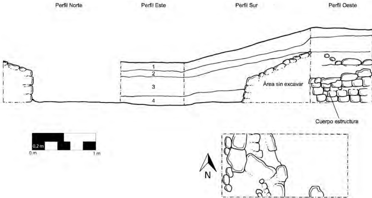
Figura 10.10 Perfiles y planta de la unidad CR120A-6 (Dibujo y calco por A. Roche)
