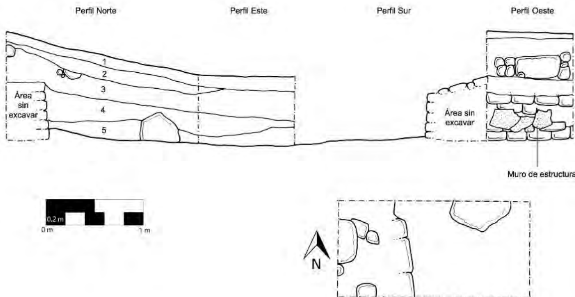
Figura 10.5 Perfiles y planta de la unidad CR120A-3 (Dibujo y calco por A. Roche)
