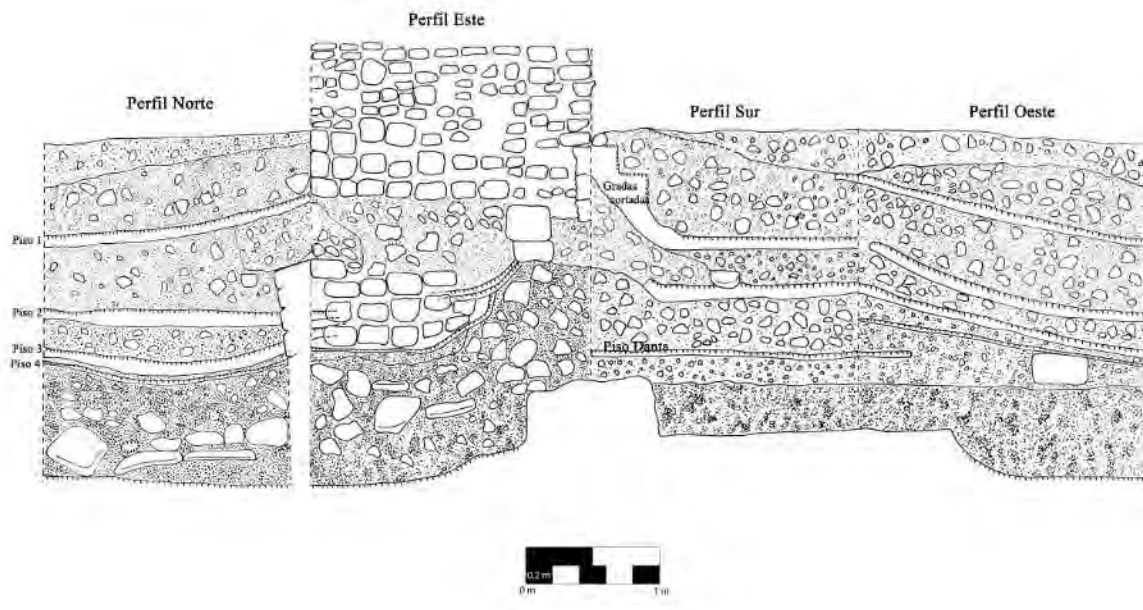
Figura 7.23. Perfiles de la excavación dentro de la Estructura 13Q-2-Sub1, unidad CR32H-19 (Dibujo por E. Gómez)
