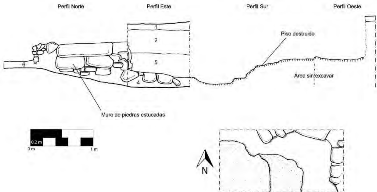
Figura 9.3 Perfiles y planta de la unidad CR116-2 (Dibujo y calco por A. Roche)
