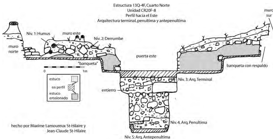
Figura 5.9. Perfil interior Este de la Unidad CR20F-8. Cuarto Norte, Estructura 13Q-4F (Dibujo por M. Lamoureux St-Hilaire)
