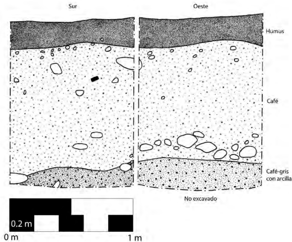
Figura 14.17. Perfil de la Unidad CAR-12A-2 (Dibujo y calco por D. Chatelain).
