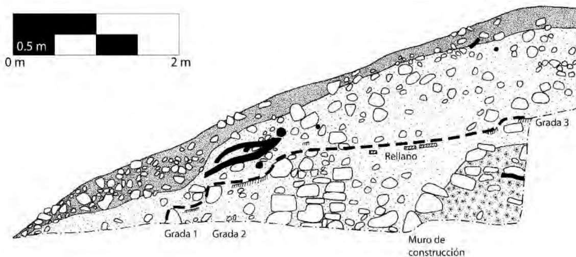
Figura 14.13 Perfil oeste de la trinchera de saqueo de Estructura A-4, Unidad CAR-1B-2 (Dibujo y calco por D. Chatelain).
