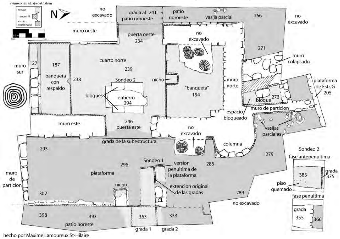
Figura 5.7 Planta de la Unidad CR20F-8. Cuarto Norte de la Estructura 13Q-4F (Dibujo por M. Lamoureux St-Hilaire)
