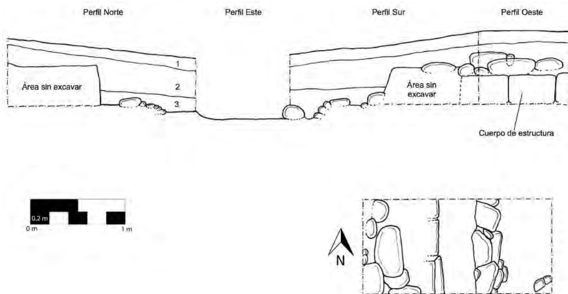
Figura 10.3 Perfiles y planta de la unidad CR120A-1 (Dibujo y calco por A. Roche)
