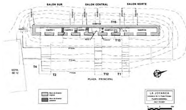
Figura 15.32 Estructura 5E-13 del sitio La Joyanca (Arnauld y Arredondo 2002). Edificio largo de carácter administrativo y de dimensiones similares a la Estructura 5 de Las Guacamayas.
