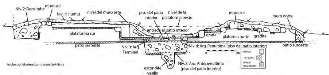
Figura 5.18. Perfil oeste de la Unidad CR20I-1, Estructura 13Q-4I (Dibujo por M. Lamoreux St-Hilaire)
