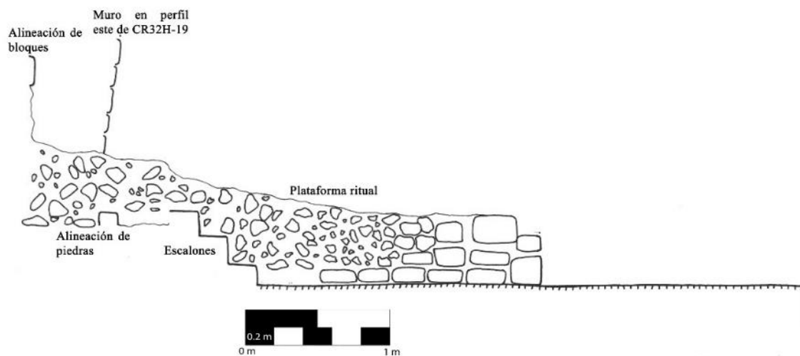
Figura 7.7 Corte Este-Oeste, mostrando entre otros, los escalones, asociados a la penúltima etapa constructiva (13Q-2-Sub3), localizados en el sector norte de las excavaciones (Dibujo por E. Gómez)
