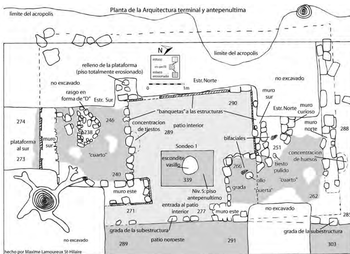
Figura 5.17. Planta de la unidad CR20I-1, Estructura 13Q-4I (Dibujo por M. Lamoureux St-Hilaire)
