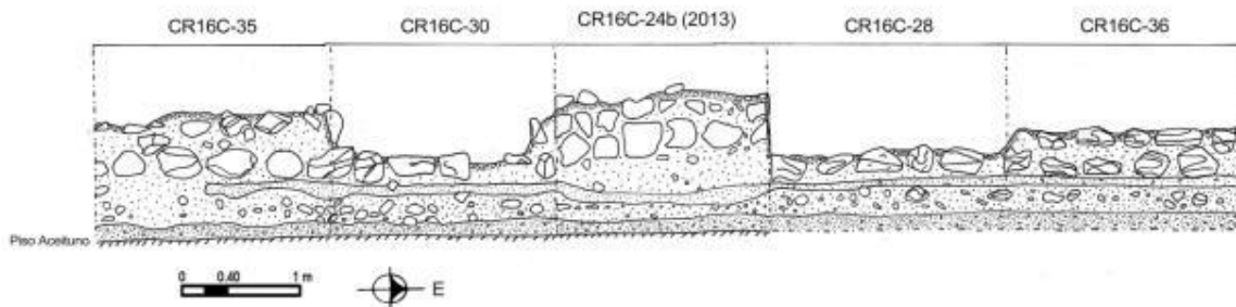
Figura 8.15 Fachada Sur del muro asociado al Piso Aceituno (Dibujo por L. Auld-Thomas y J. Ponce)
