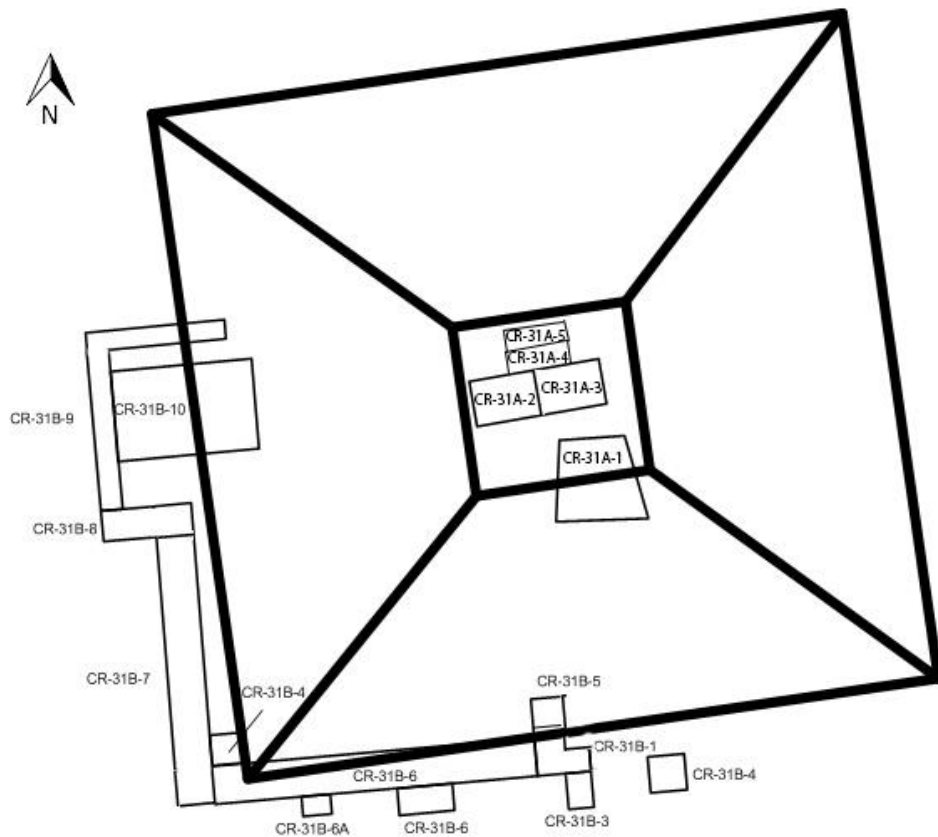
Figura 6.1 Plano de la Estructura 13Q-1 y ubicación de las excavaciones (Mapa por E. Bustamante)
