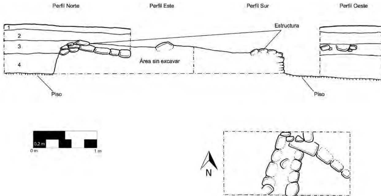
Figura 9.6 Perfiles y planta de la unidad CR116-4 (Dibujo y calco por A. Roche)
